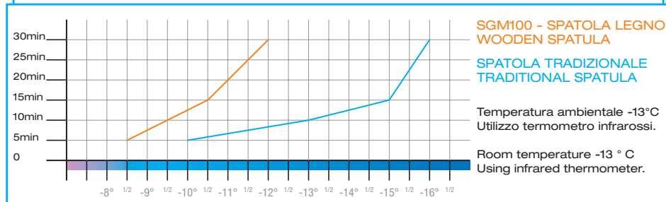
Misura temperatura manico spatole gelato - Temperature of the handle ice cream spatula.
